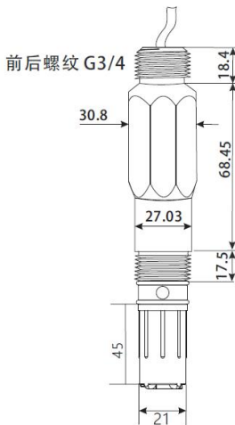
图 1 产品尺寸图 (单位: mm)
