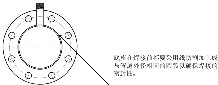
图 5 理想底座焊接位置
