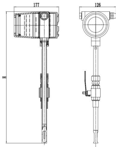
图 2 插入式外形尺寸图（单位：mm）
