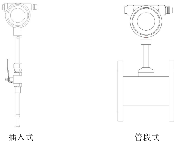
图 1 热式气体质量流量计产品分类
