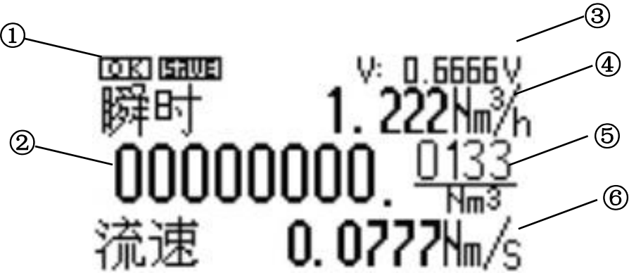
图 8 主界面
