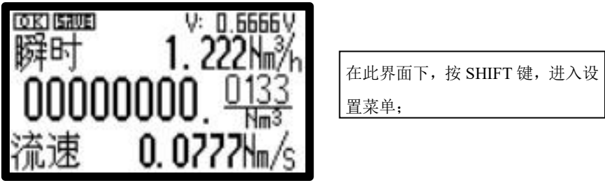
图 9 主界面
