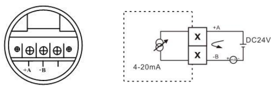
图 3-2 A 型转换器接线图
