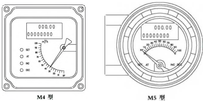
图 20 指示器示意图
