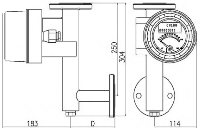
图 17 标准型 M5 指示器
