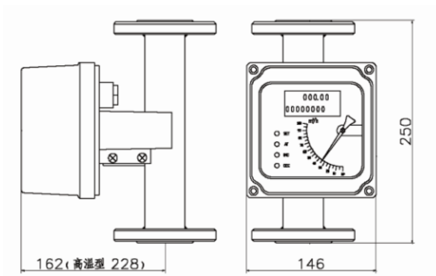
图 2 标准型 M4 指示器
