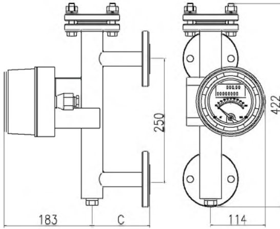
图 15 标准型 M5 指示器
