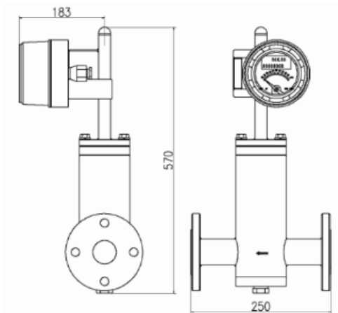
图 9 T 型结构 M5 指示器
