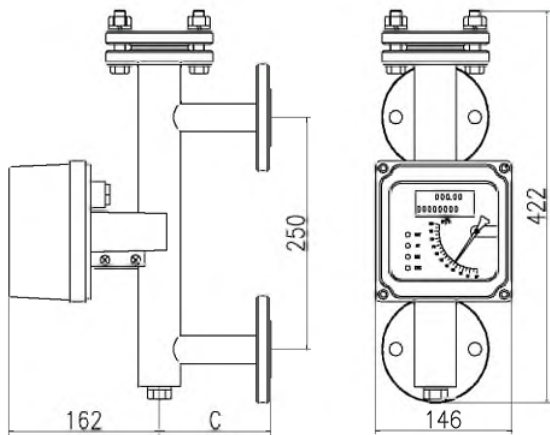
图 14 标准型 M4 指示器
