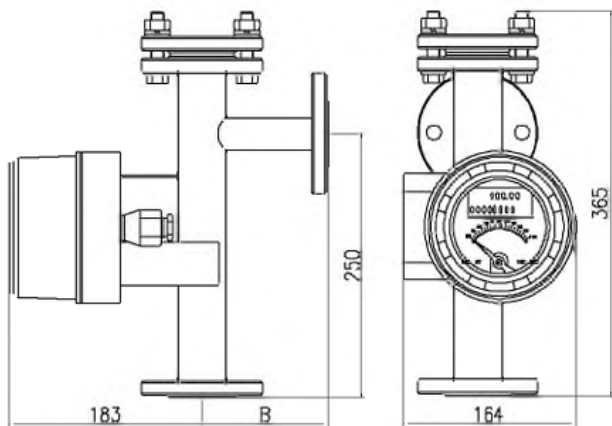
图 13 标准型 M5 指示器
