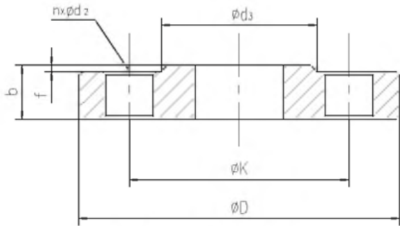
图 18 法兰外型尺寸
