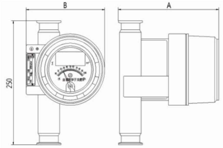
图 7 卫生型 M5 指示器
