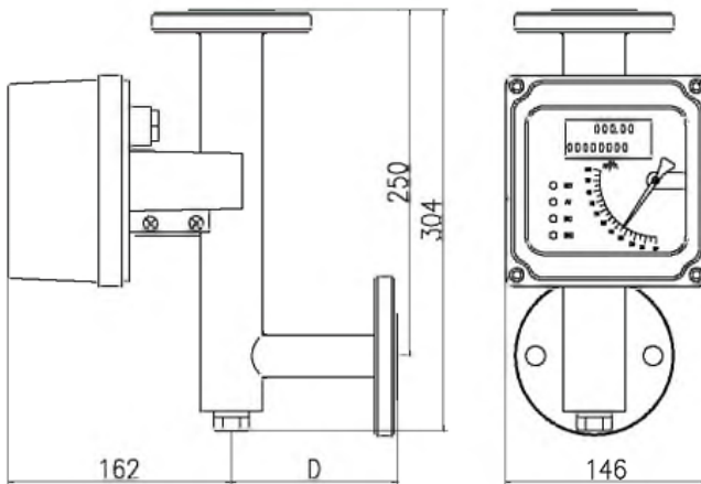
图 16 标准型 M4 指示器
