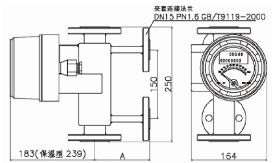
图 5 冷却夹套型 M5 指示器
