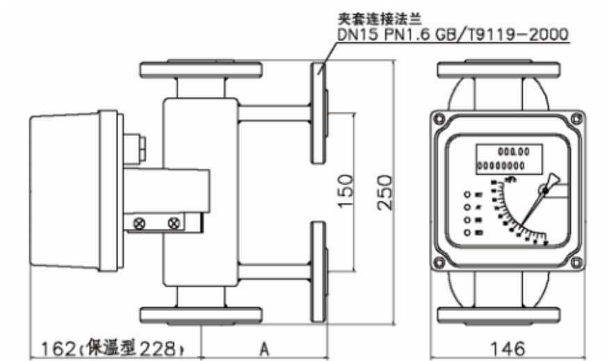
图 4 冷却夹套型 M4 指示器
