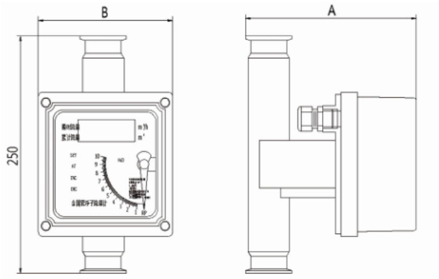
图 6 卫生型 M4 指示型
