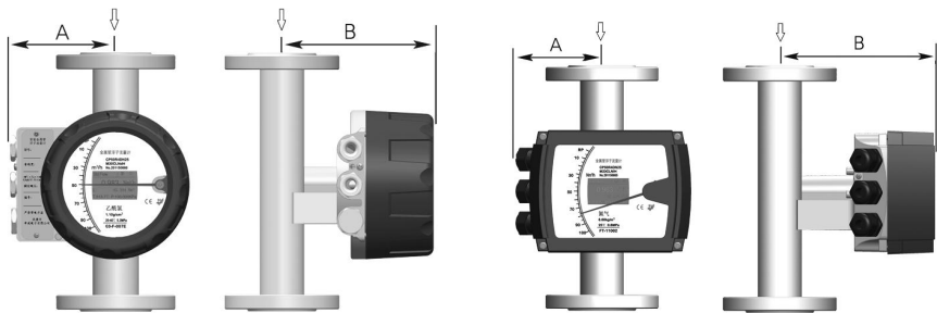
上进下出型配 M30/M20 指示器外形尺寸及重量表
