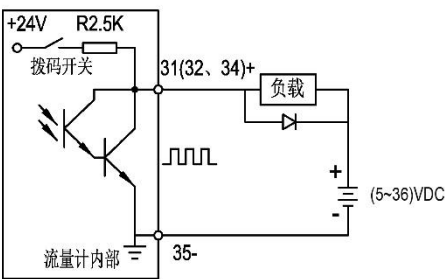
脉冲、批次、报警无源输出接线 (拨码开关处于OFF)
