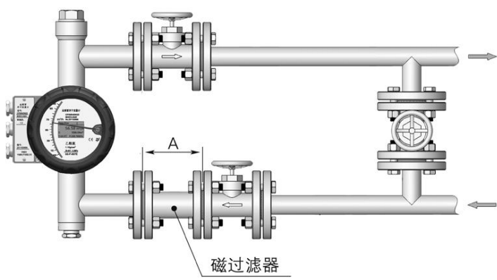
图 8 下横进上横出型安装图
