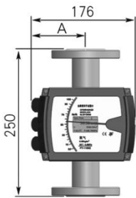
c、下进上出型标准型及夹套型配 M20 指示器外形尺寸及重量表
