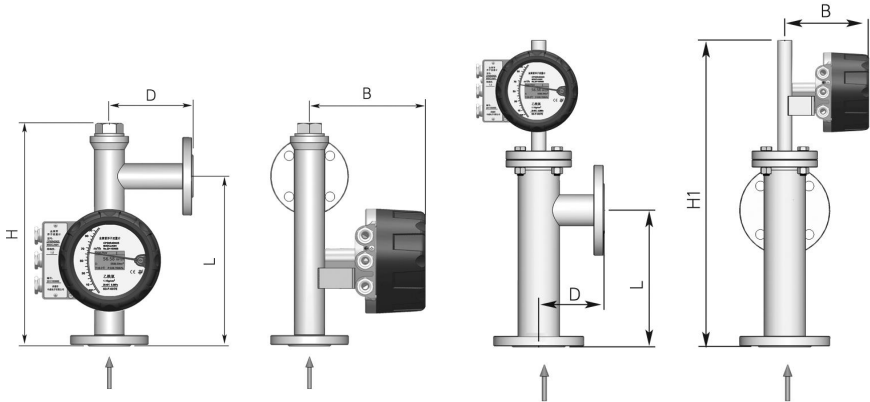
图 16 DN15 ~ DN25( 标准型 ) 图 17 DN50 ~ DN200( 标准型 )
