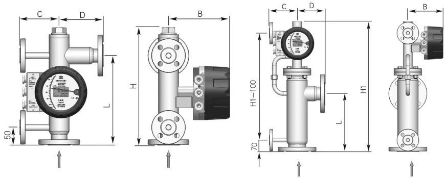
图 18 DN15 ~ DN25( 夹套型 ) 图 19 DN50 ~ DN200( 夹套型 )
