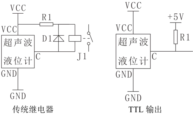
图 16 NPN 输出接线
