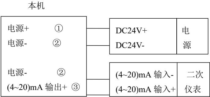
图 14 三线制液位计与二次仪表连接
