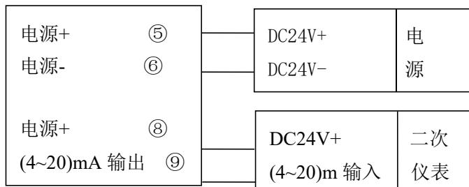
图 12 四线制液位计与二次仪表连接
