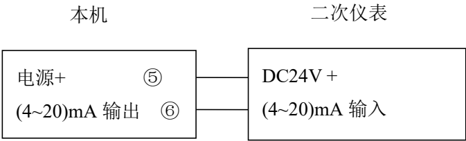
图 10 二线制液位计与二次仪表连接
