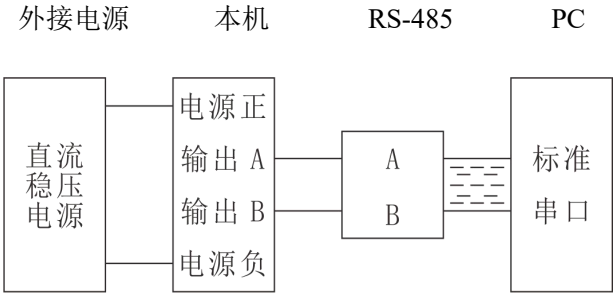
图 15 串口输出接 PC
