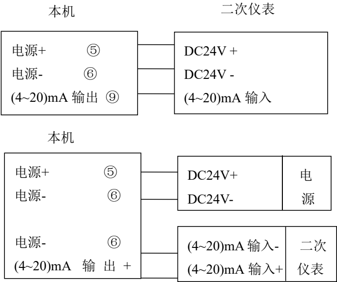
图 11 三线制液位计与二次仪表连接
