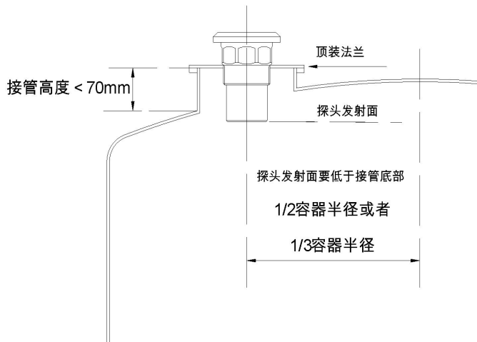
图 9 安装在法兰上--拱形罐顶
