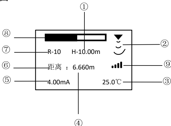
图 26 监控界面
