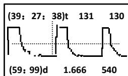
图 50 波形显示界面
