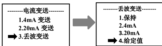
图 35 丢波变送设置界面
