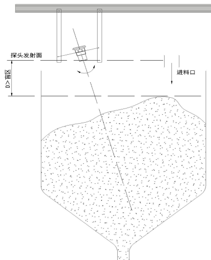
图 15 龙门框安装
