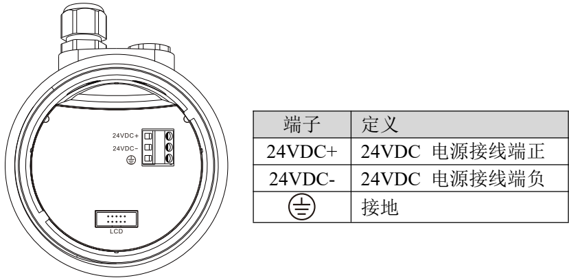
图 21 一体式二线制端子说明
