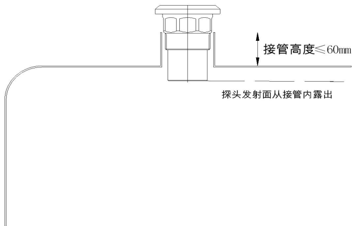
图 7 探头安装在螺纹接管上
