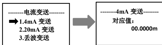
图 34 4mA 变送设置界面
