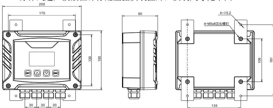
图3 分体式主机安装尺寸（单位：mm）
