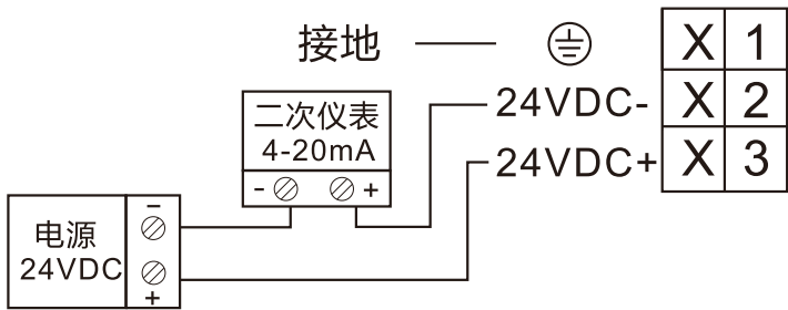
图 22 一体式二线制接线示意图
