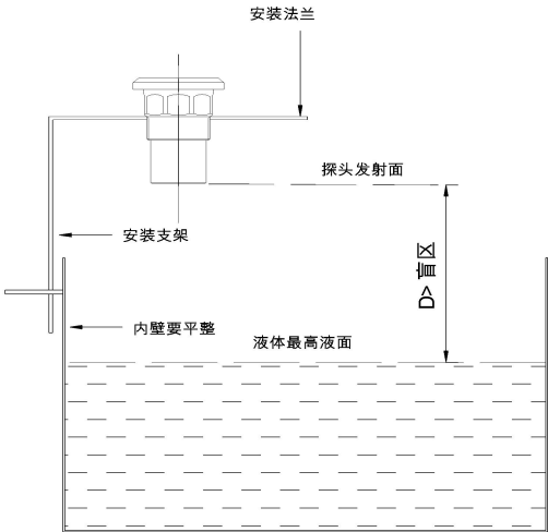
图 10 开口容器上--顶部靠一侧支架安装在开口容器上安装，可以把传感器安装在容器的正中间。
