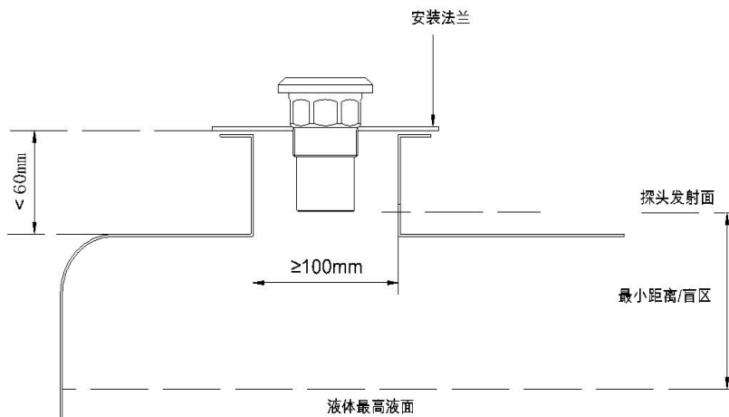
图4 法兰安装--安装在很短的接管内
