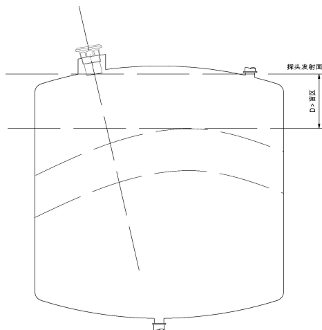
图 14 螺纹接管安装
