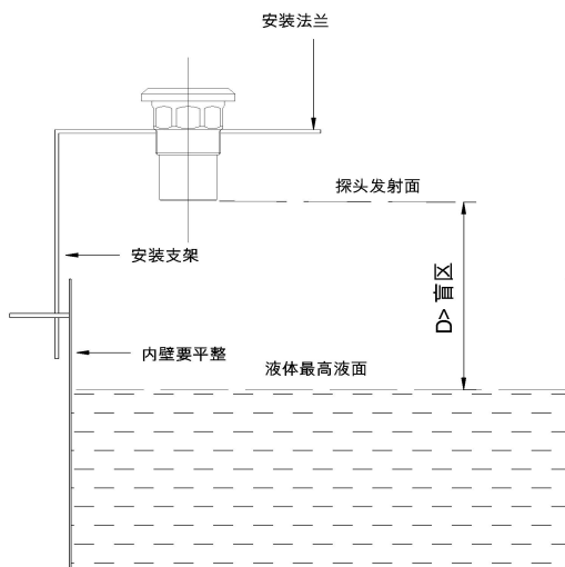
图 11 开口容器上--顶部居中支架安装
