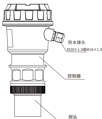
图 1 一体式超声波液位计结构示意图
