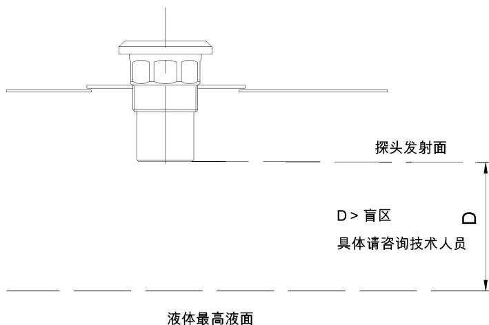
图 6 法兰型安装在无接管平顶罐上
