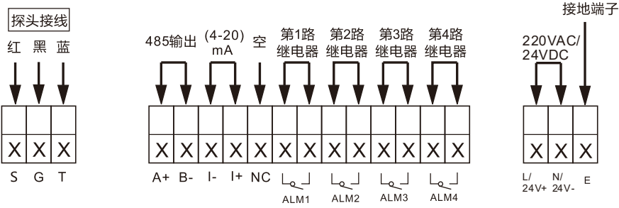
图 24 分体式接线端子示意图 表 7 分体式端子定义
