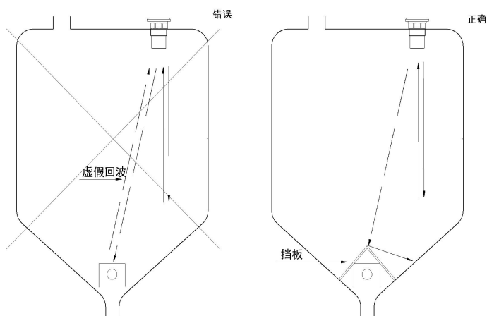
图 18 容器底部有平顶的凸起物--要加折射板
