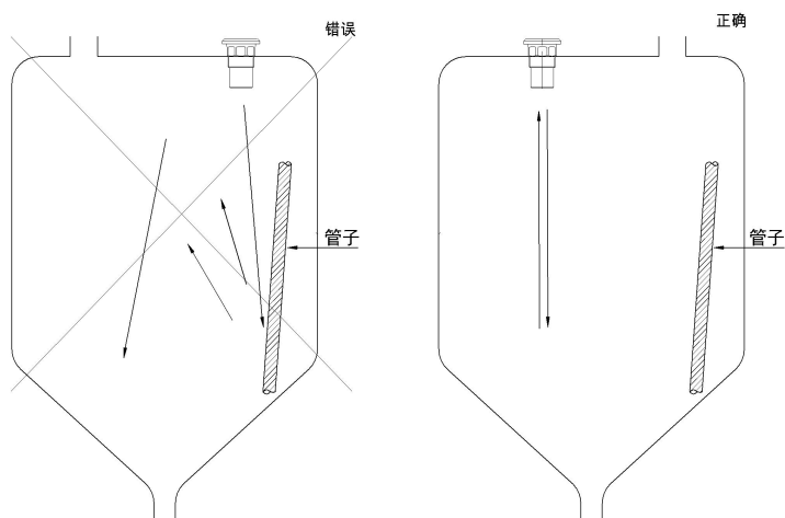
图 19 容器内有障碍物管子--要远离管子一定距离
