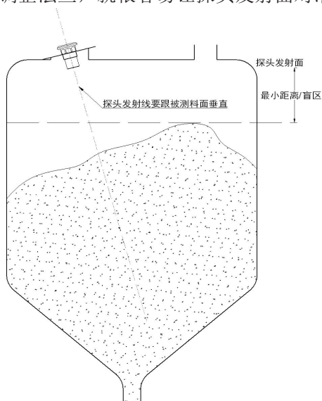
图 13 安装在容器法兰上
