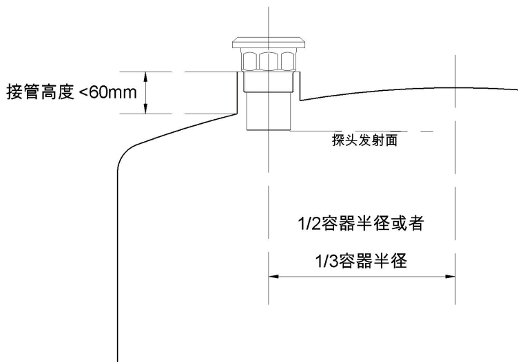
图 8 安装在螺纹接管上--拱形罐顶
