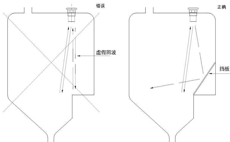
图 17 容器内台阶样的障碍物--需要加斜的横板把虚假回波折射走 如果容器下部有物体的上表面是平面，必须用一定角度的折射板挡上。
