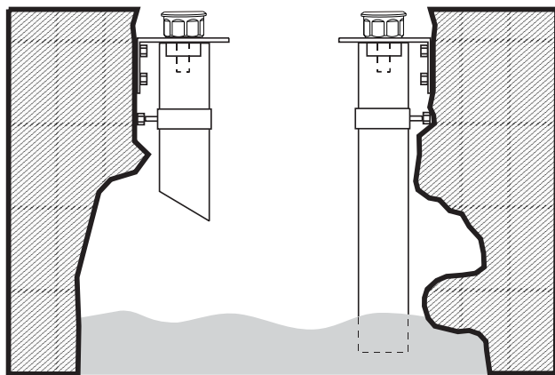
图 12 接管和测量套管用于排水井测量
