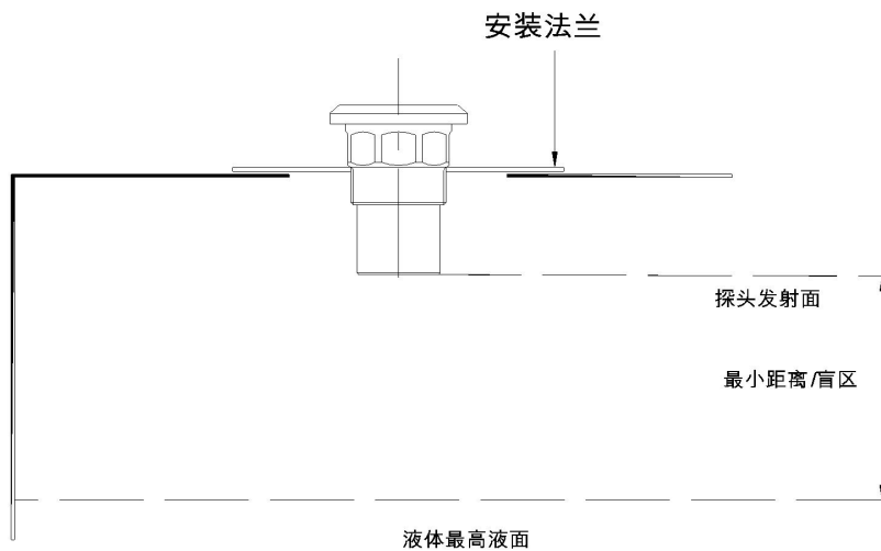
图5 法兰型（锁紧法兰）--安装在平顶罐上
