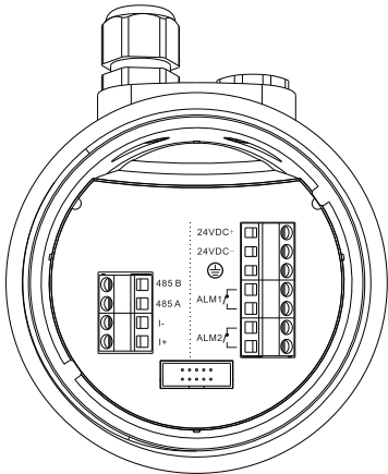
图 23 一体式四线制接线端子示意图
