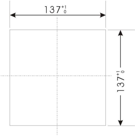
图 89 仪表开孔尺寸
