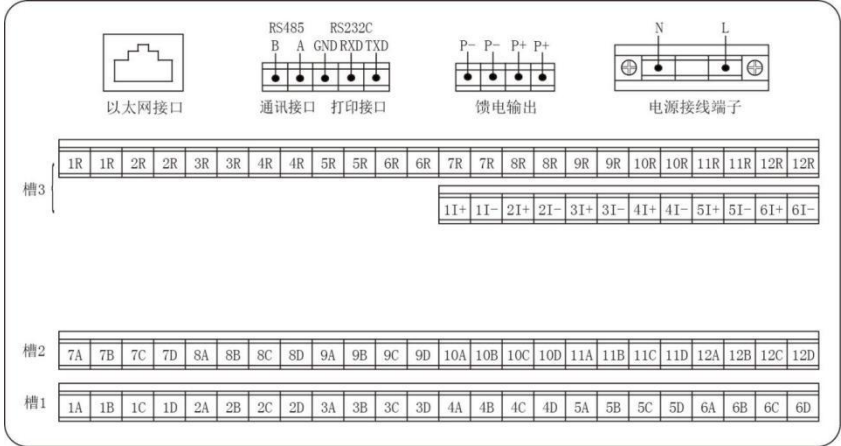
配线说明
