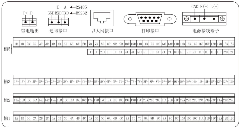
配线说明
