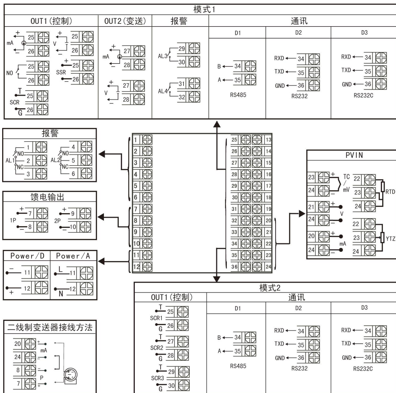
图 2 规格尺寸为 A、B、C 型接线图
