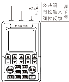
图 7 调节阀门
