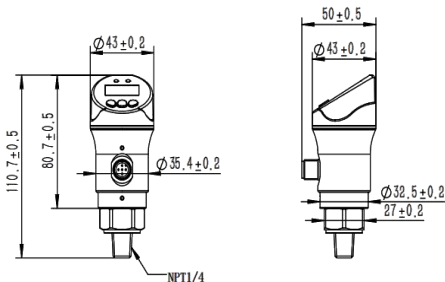
图 4 产品外形尺寸图（NPT1/4 螺纹）
