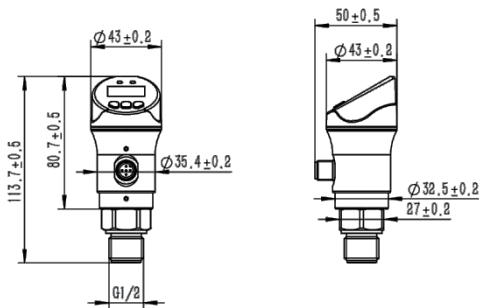
图 1 产品外形尺寸图（G1/2 螺纹）
