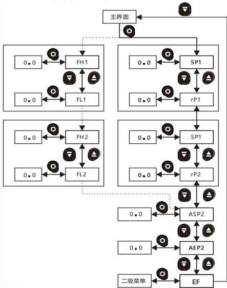
图 14 一级菜单设置流程图
