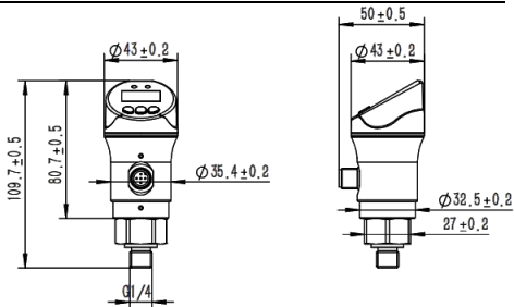
图 2 产品外形尺寸图 (G1/4 螺纹)
