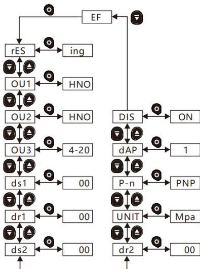
图 15 二级菜单设置流程图
