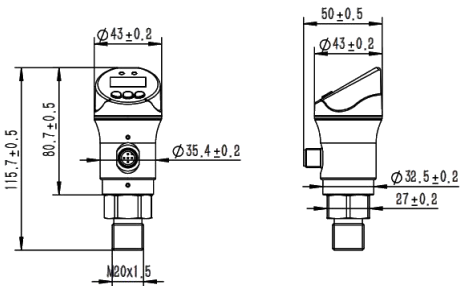
图 3 产品外形尺寸图 (M20×1.5 螺纹)
