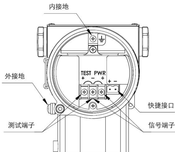
图 12 电气连接图
