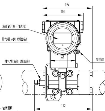
图 8 水平配管连接方式 (正面)
