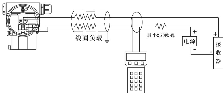
图 11 HART 通讯连接图
