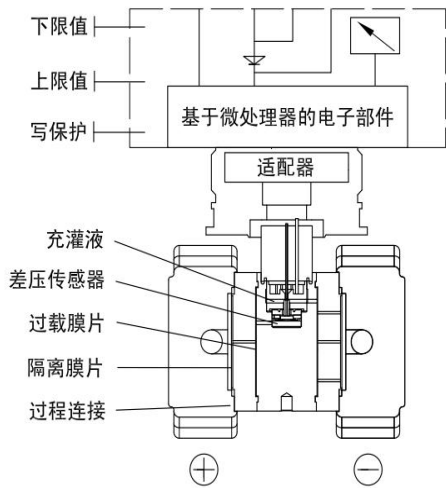
图 2 差压变送器
