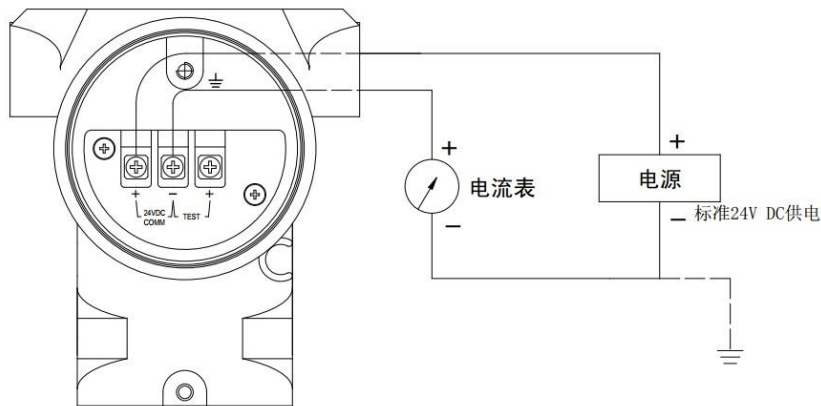
图 4 电气接线图
