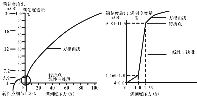
图 4 方根输出曲线
