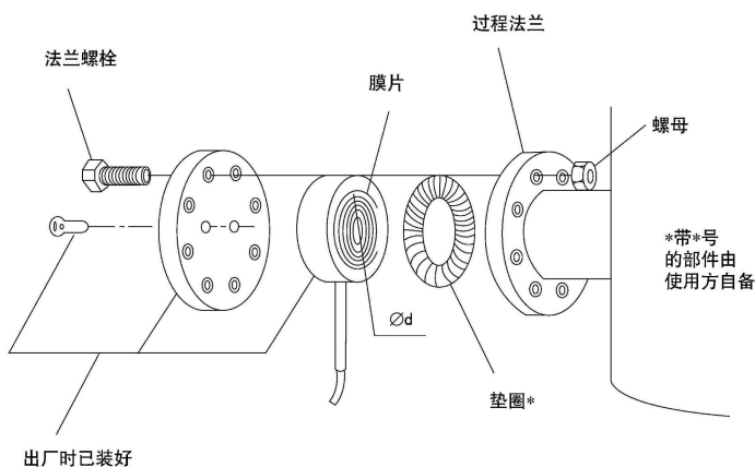
图 21 远传法兰隔膜密封部位的安装
