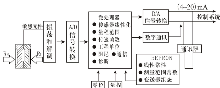
图 1 工作原理
