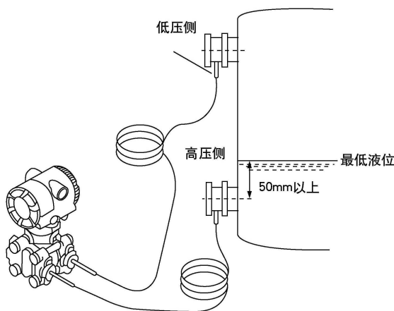
图 22 液罐安装实例
