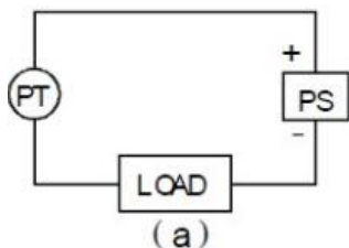
图 1-3a 非接地系统
