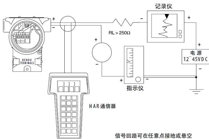
图 16 智能变送器外部电路接线图
