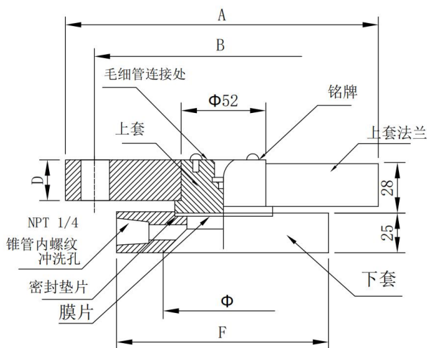
图 12 RFW 型法兰安装远传装置外形尺寸图
