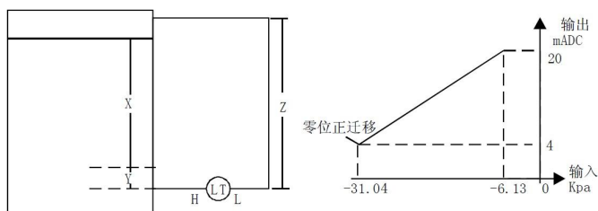
图 18 密闭容器导压链接测量举例
