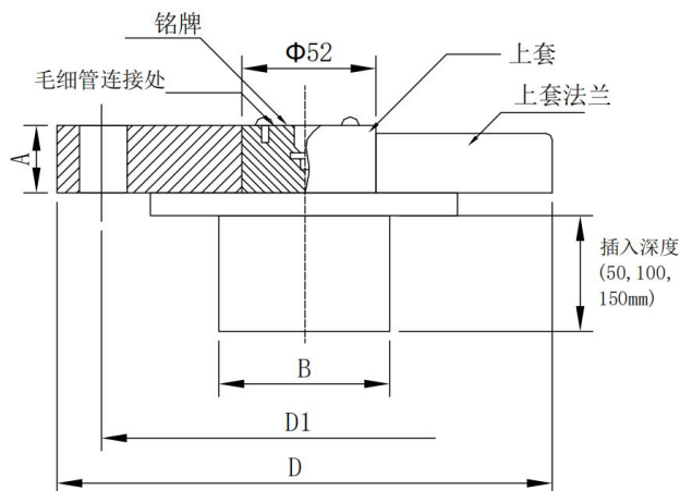
图 11 EFW 型插入式远传装置外形尺寸图 (尺寸见表 1)
