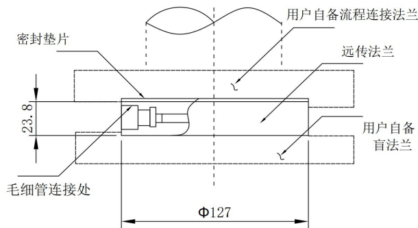
图 10 PFW 型扁平式远传装置外形尺寸图
