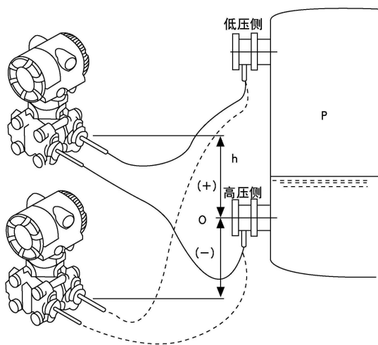
图 23 在罐体安装位置实例
