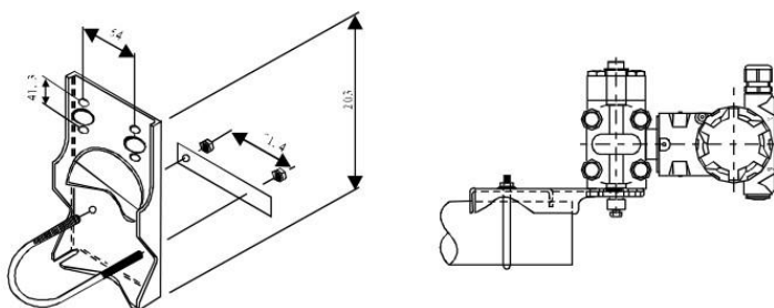
管装平支架 B3
