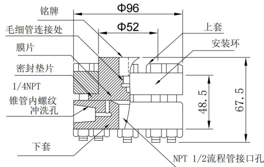
图 9 RTW 型螺纹安装式远传装置外形尺寸图
