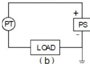
图 1-3b 电源负端和负载之间接地
