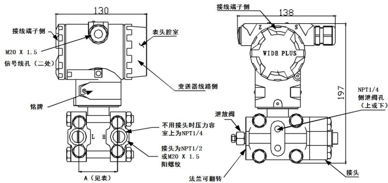
图 7 一般变送器外形图
