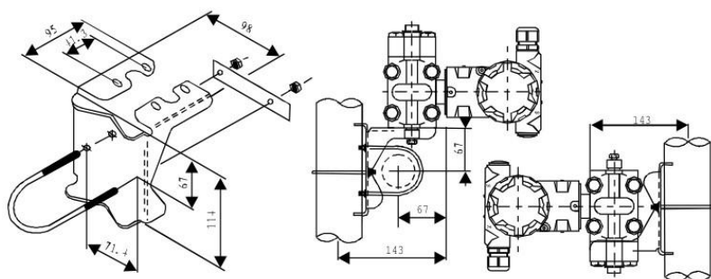
管装弯支架 B1
