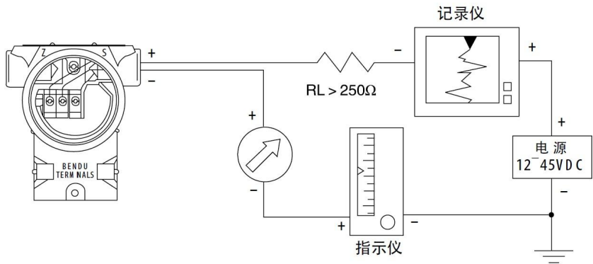
图 15 非能变送器外部电路接线图
