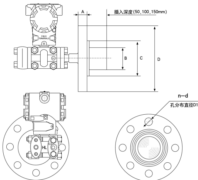
图 8 法兰液位安装示意图
