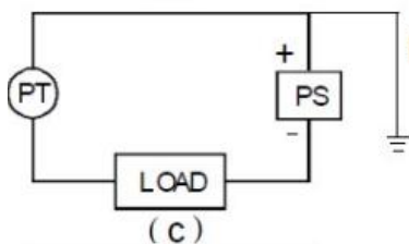
图 1-3c 变送器的正端和电源之间接地
