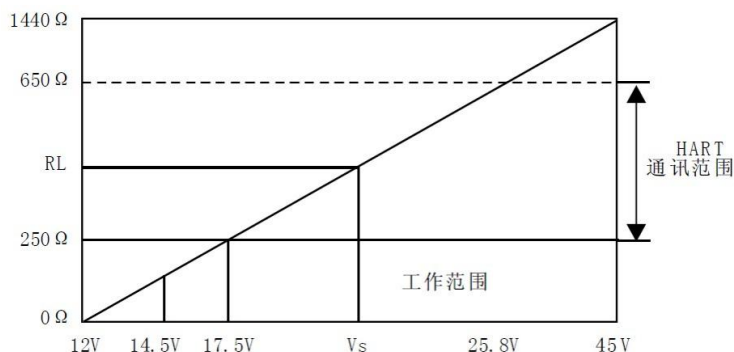
图 5 负载特性图
