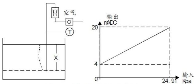
图 19 吹气法测量液位举例
