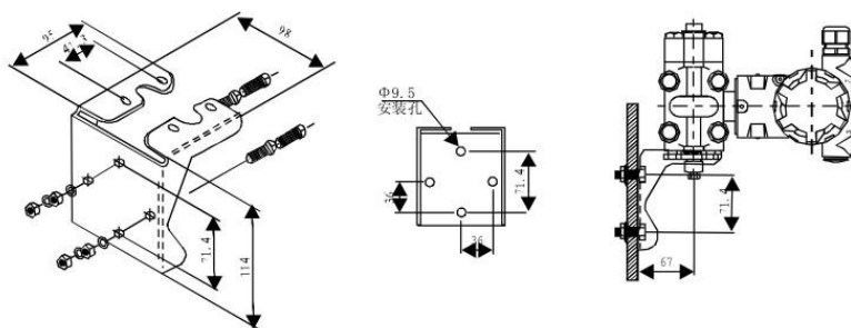
盘装弯支架 B2
